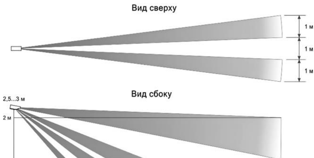
Рисунок 1.1 - Форма зоны обнаружения
